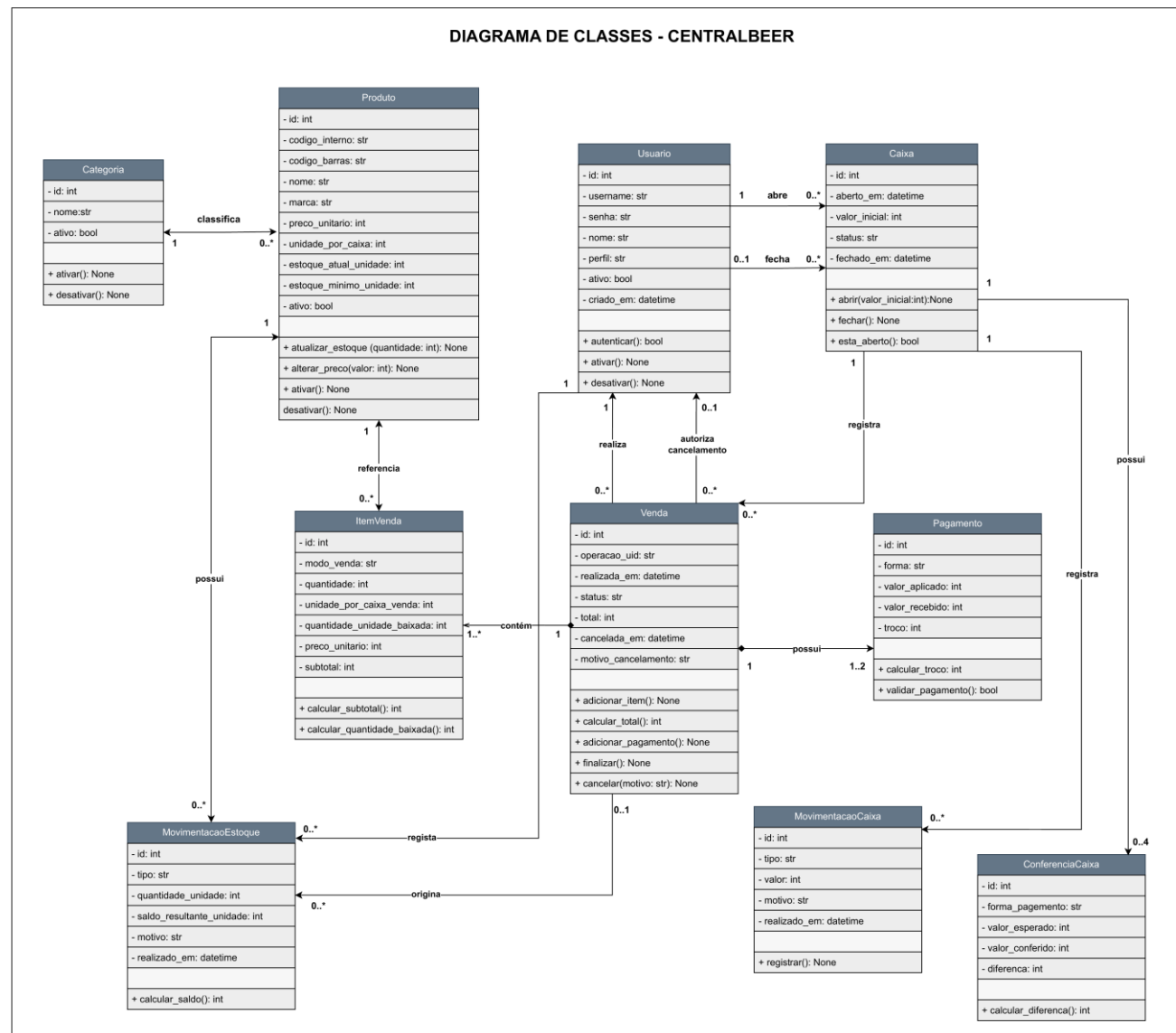
Figura 1 - Diagrama UML de classes do CentralBeer. Fonte: elaboração própria em diagrams.net (2026).
